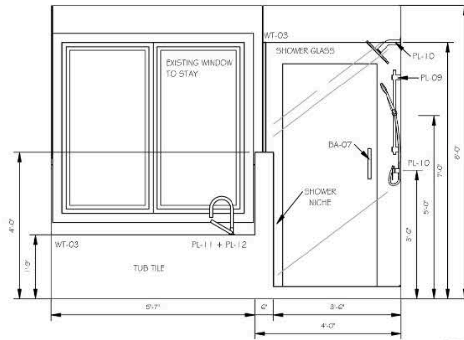
3 ENSUITE TUB WALL SCALE: 3/8" = 1'-0"
