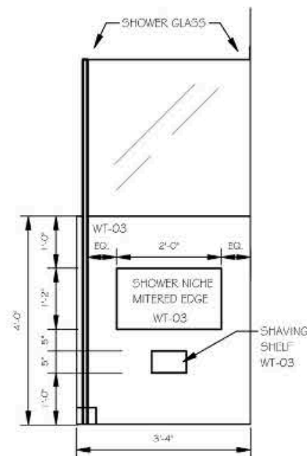
4 ENS. NICHE WALL SCALE: 3/8" = 1'-0"
